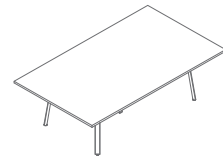
PLF25 2400 / 1400 / 740 81 kg
