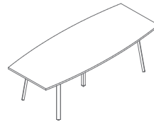
PLF24 2400 / 800-1000 / 740 58.3 kg
