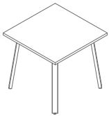
PLF81 800 / 800 / 740 21.5 kg
