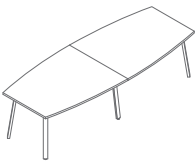
PLF18 2000 / 1100-800 / 740 78,5 kg
