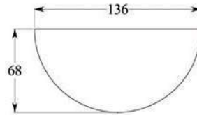
demi-lune 68 x 136 cm 68x136cm extension unit CITU63
